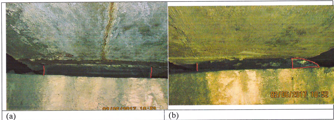
Figura 40: (a) neoprene, (b) aparelho de apoio com resíduo de concreto impedindo movimento;
