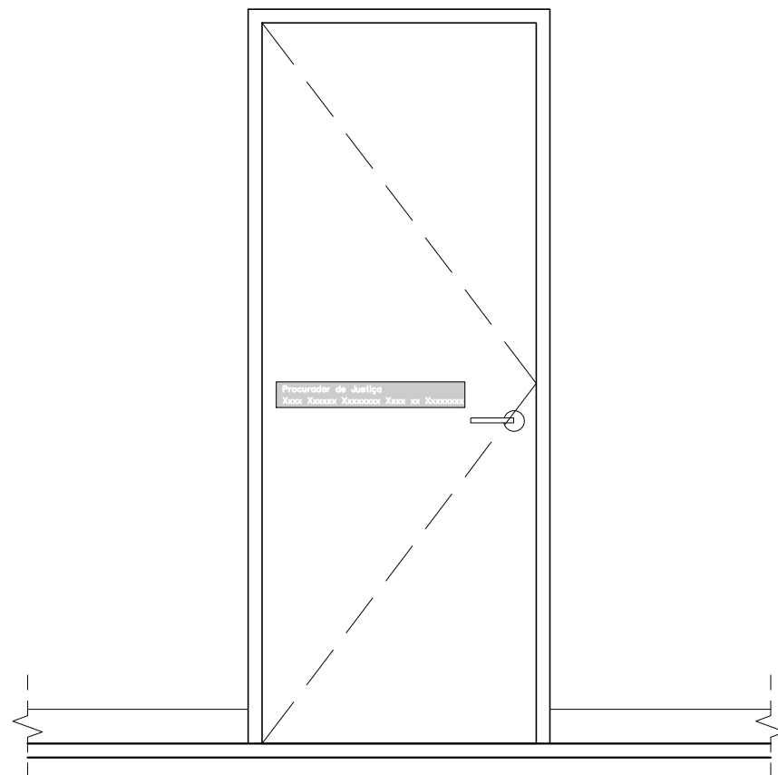
2 EXEMPLO DE APLICAÇÃO DA CHAPA DE AÇO escala : SEM ESCALA
