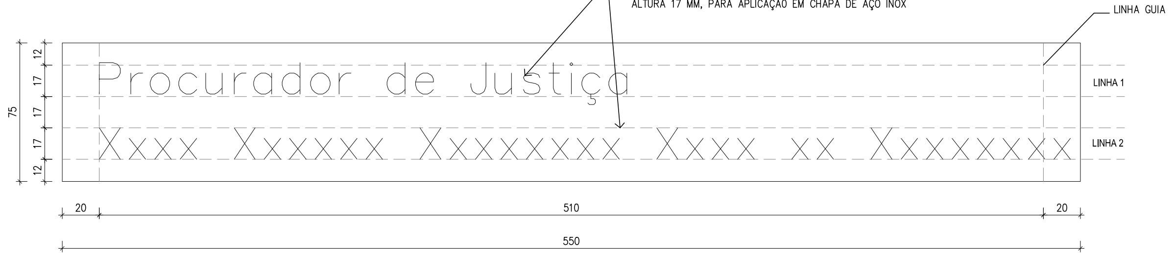
1 DETALHAMENTO DE ADESIVO PARA CHAPA DE AÇO escala : SEM ESCALA
