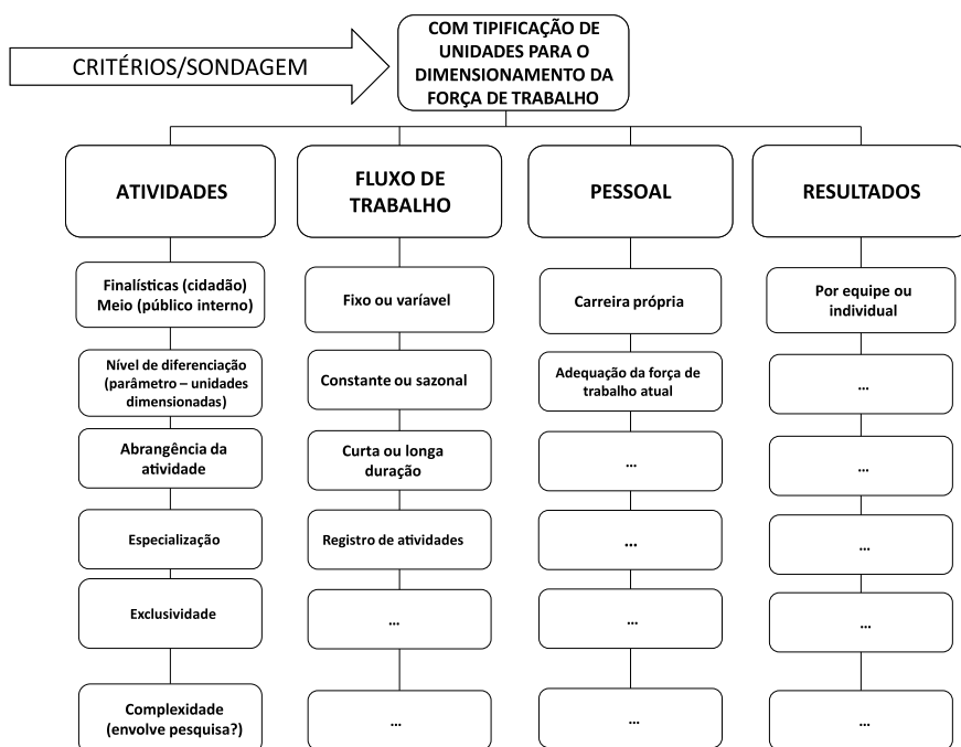
Figura 3.4 – Famílias de critérios para o DFT com tipificação
