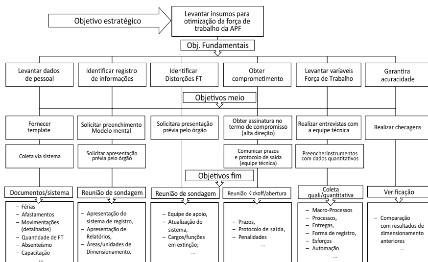
Figura 3.3 – Hierarquia de objetivos relativos ao DFT com base na aplicação da abordagem VFT
