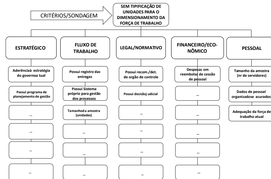
Figura 3.5 – Família de critérios para o DFT sem tipificação
