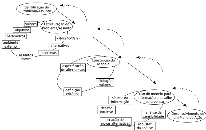
Figura 3.2 – Etapas do processo de análise de decisões considerando a abordagem AMD
