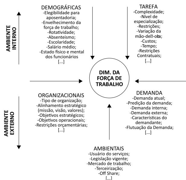
Figura 3.1 – Variáveis importantes para o DFT
