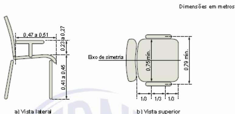
Figura 27 – Dimensões para assentos para pessoas obesas
