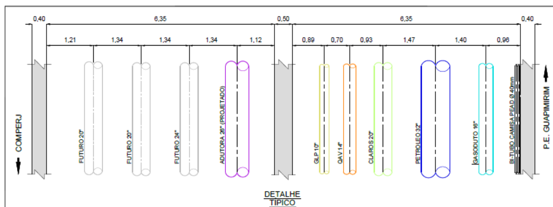
Figura 6 – Vista superior da travessia sobre o rio Macacu.
