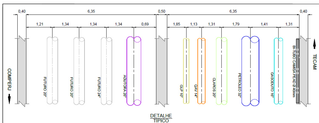
Figura 5 – Vista superior da travessia sobre o rio Guapiaçu.
